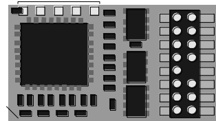
Programmierpads, Kontaktierung verboten! MX630P (mit PluX16)
